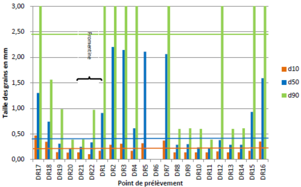
Illustration 24 : Comparatif des caractéristiques granulométriques des matériaux prélevés lors du dragage du chenal en juin 2011 par le Conseil Général de Vendée avec celles du sable de la plage de la Tonnelle (Renault, BRGM, 2011)
