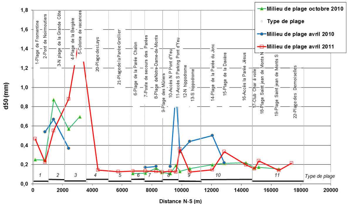
Illustration 10 : Variation du d50 du nord vers le sud en milieu de plage. Comparatif 2010/2011 (Renault, BRGM, 2011)
